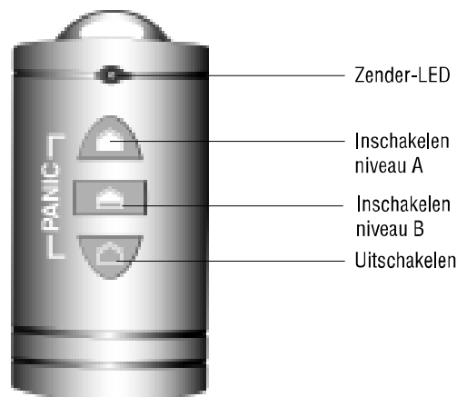
Afb. 2. 725r Afstandsbediening.
